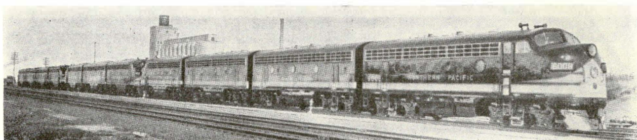
Tre sammenkoblede General Motors-diesellokomotiver på Northern Pacific Railroad. — Det forreste og det bageste er godstogslokomotiver bestående af fire enheder, som stort set er mage til DSB's nye diesellokomotiv og har samme 16-cylindrede motor. Det mellemste er et eksprestogslokomotiv bestående af tre enheder, formentlig med to motorer af den tilsvarende 12-cylindrede model.
